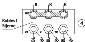
Klemmerække kobles således til 2,5 KW.
