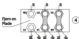
Klemmerække kobles således til 5 KW.
