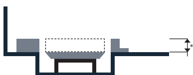
Tværsnit af afløbsarmatur med ramme/ med Custom (med eget materiale monteret).
