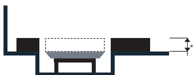
Tværsnit af afløbsarmatur uden ramme/ med Custom (med eget materiale monteret).
