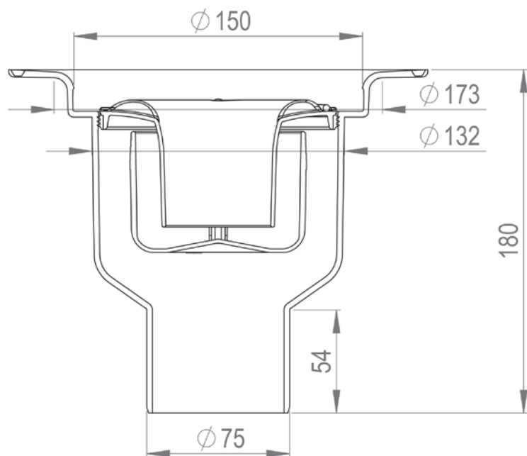
Tilbehør: VVS nr. 153479-225 indbygnings vandlås
