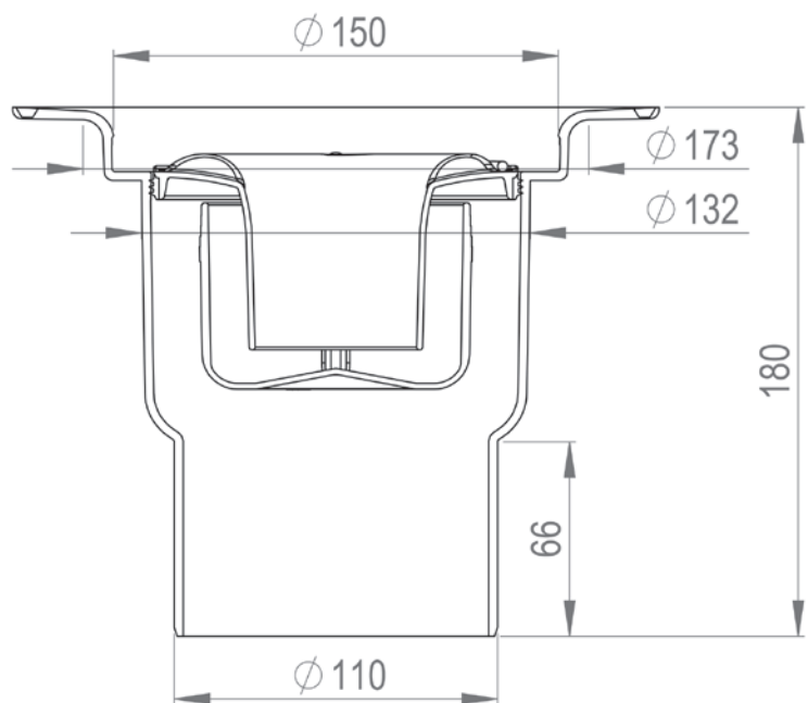
Tilbehør: VVS nr. 153479-120 indbygnings vandlås
